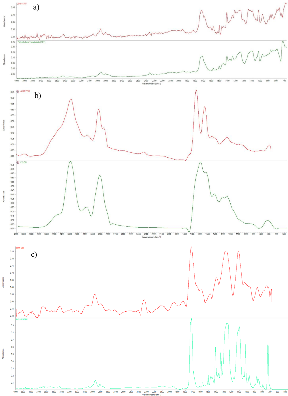
Hình 7. Một số hình ảnh phổ polymer vi nhựa thu được trong mẫu trầm tích tại vị trí ĐN1: a) PET; b) Nylon; c) Polyester.
